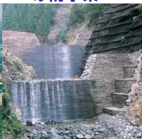
砂防事業
